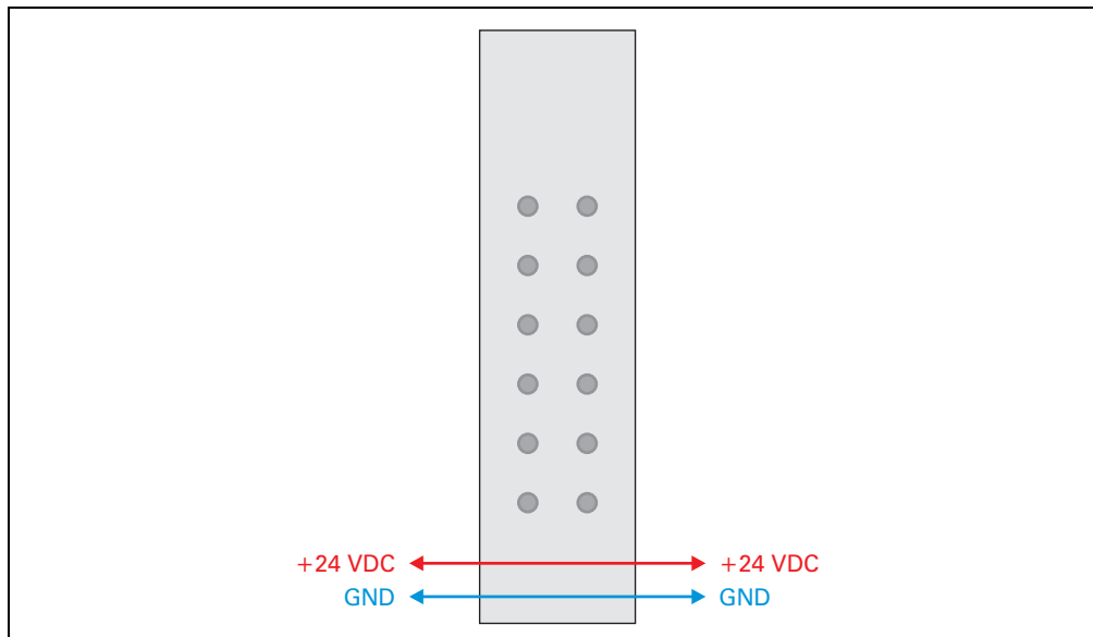
Abbildung 61: BM11 Potenzialführung
